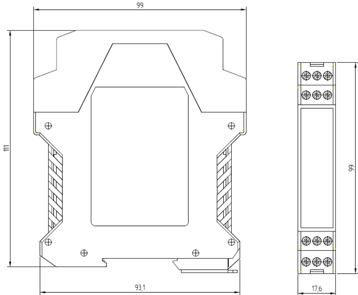
Малюнок Д.1.1 Габаритні і установочні розміри бар'єру іскрозахисту БИЗОН 2Ex.24.24
